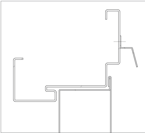
Montering på karm B (karm A), snitt B-B
