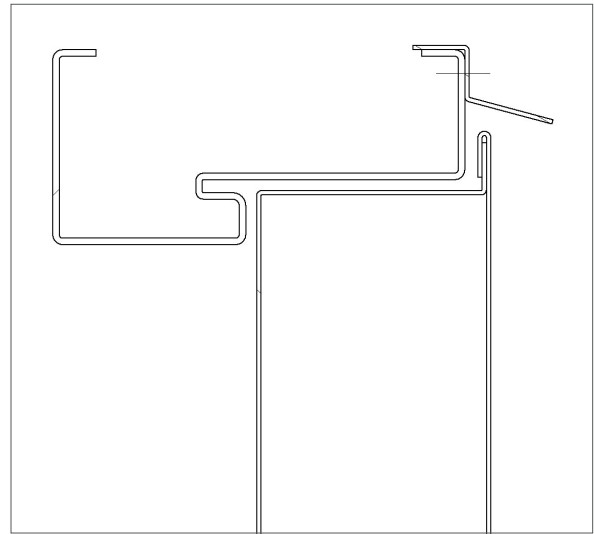
Montering på karm C, snitt B-B
