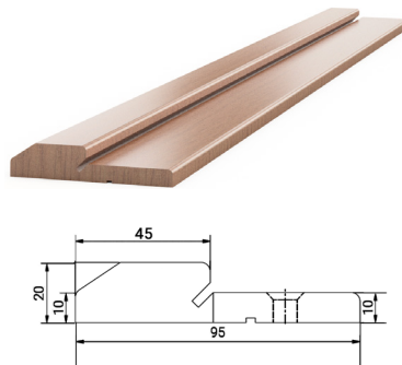
Fasad ektröskel
