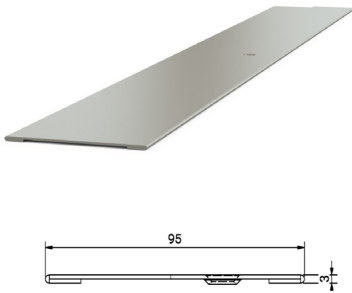
Slät tröskelplatta
