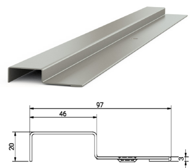
Rak anslagströskel
